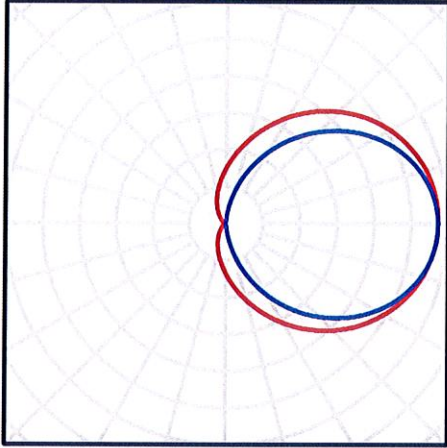
■ 配光線図（拡散）
