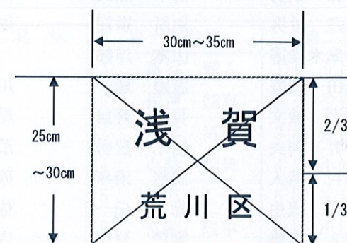
図 1 ゼッケンの縫い付け方
